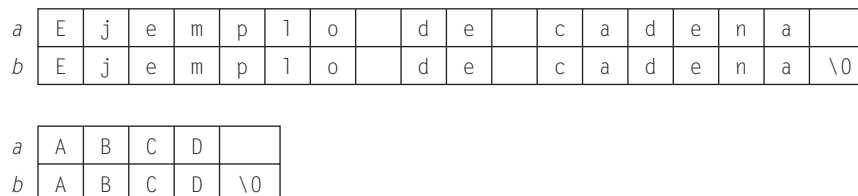
Figura 9.1. a) array de caracteres; b) cadena de caracteres.
