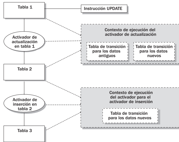
Figura 14-1 Contextos de ejecución del activador para dos activadores.
