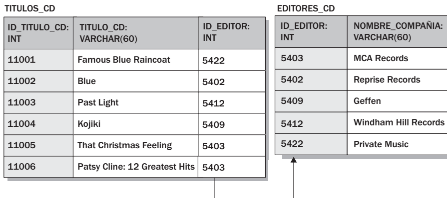
Figura 4-5 Relación entre las tablas TITULOS_CD y EDITORES_CD.
